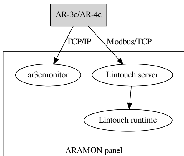
Rysunek 1: Podłączenie do rejestratora kompatybilnego z AR-3c
